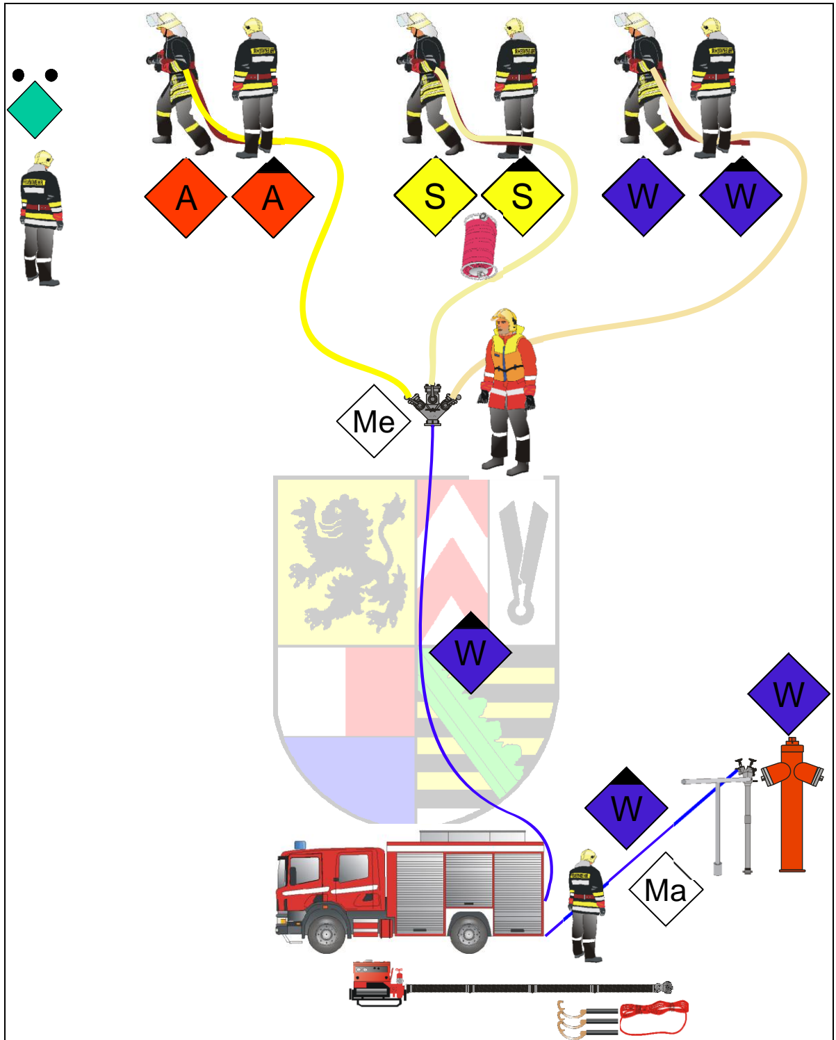
Bild 9: Löschangriff Gruppe gesamt
