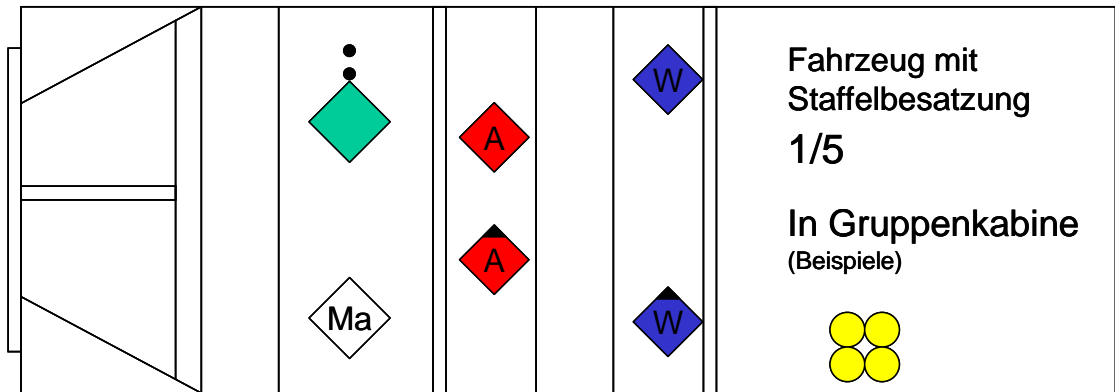
Bild 6: Sitzordnung Staffel Staffelfahrzeug
