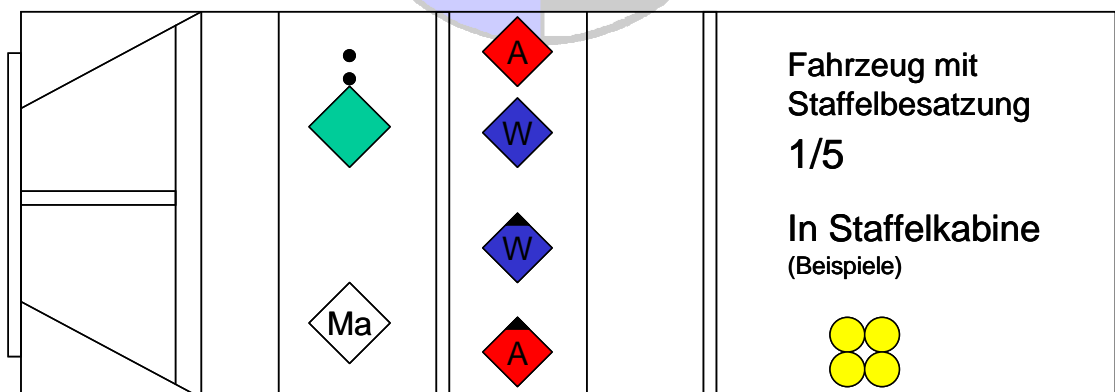
Bild 5: Sitzordnung Staffel Löschgruppenfahrzeug
