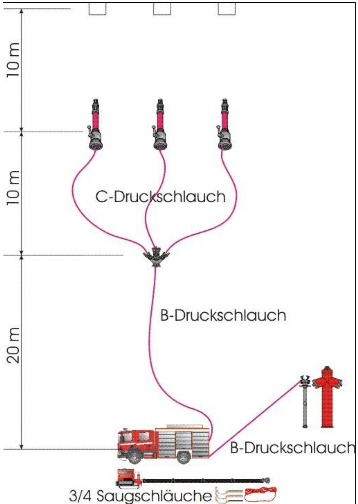
Bild 7: Aufbau Löschangriff Löschgruppe
